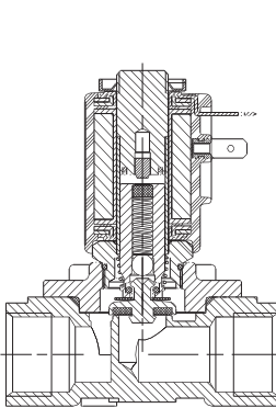
2 Way NC
