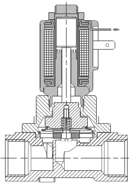
2 Way NO
