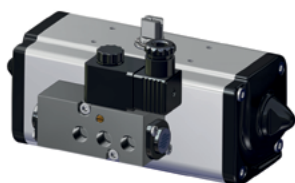
3/2 - 5/2 NAMUR הפעלה ע"י שסתום
