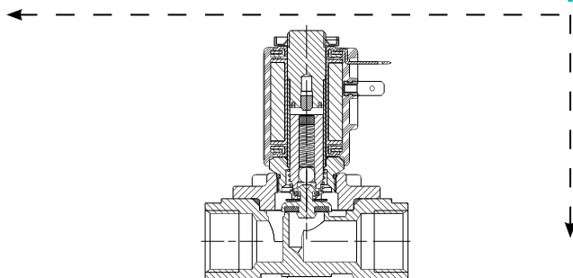
GEM-I סולנואיד פליז בקו | INLINE ד"ה: 0.8 ~ 6 מ"מ
