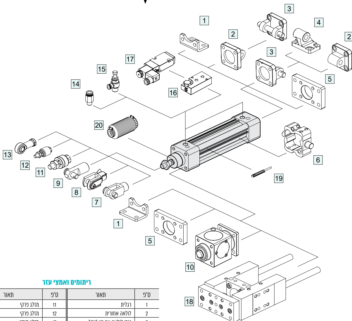
סדרה VBC/LBC גוף עגול עם מוטות קישור בקטרים 250 ~ 32 מ"מ
